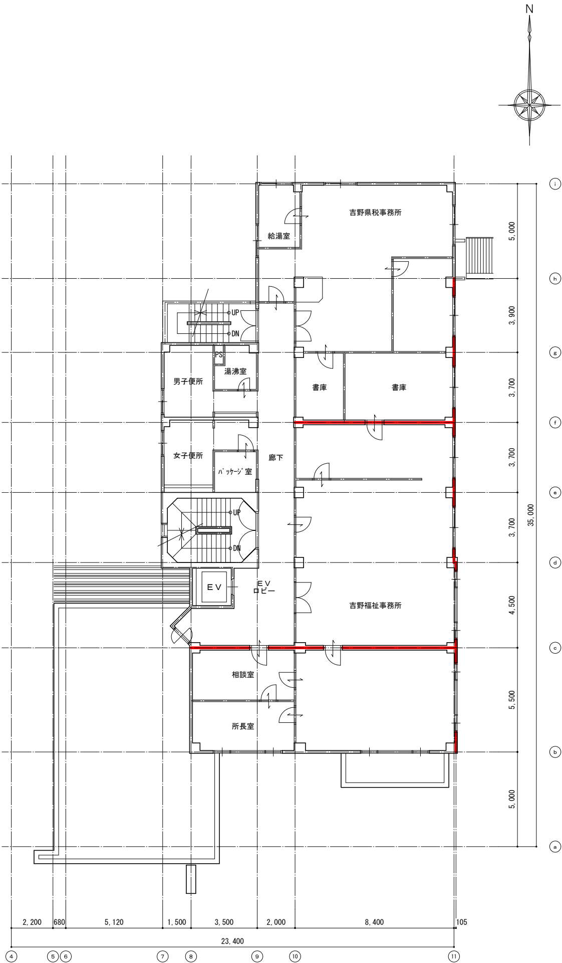
3階平面図
