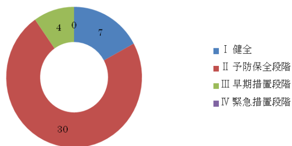
平成28年度吉野町橋梁点検結果
